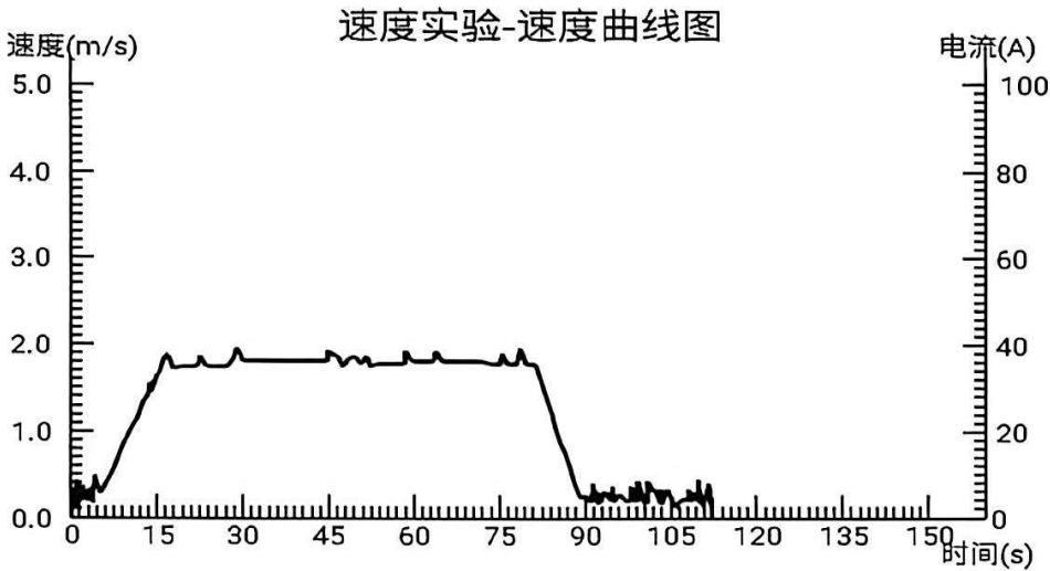
速度时间曲线
